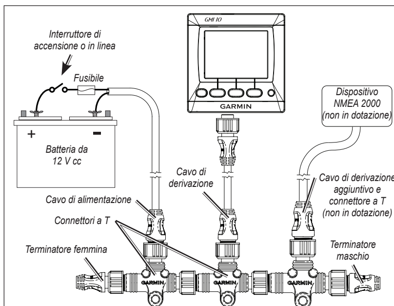
Creazione di una rete NMEA 2000 di base
