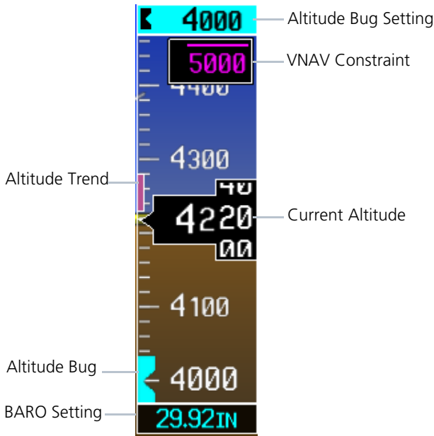
Altitude Tape
