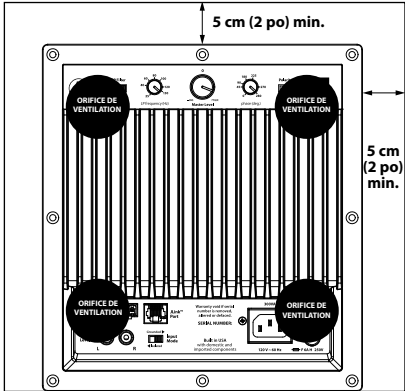
Vue arrière du boîtier :
