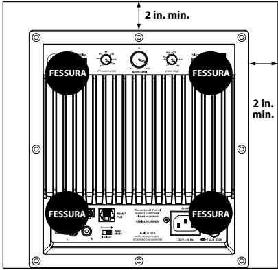
Visuale posteriore dell'installazione nella teca:
