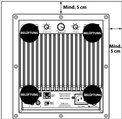
Rückansicht bei Gehäuseeinbau:
