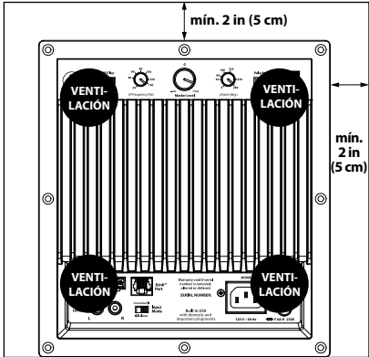
Vista trasera de la instalación en gabinete:
