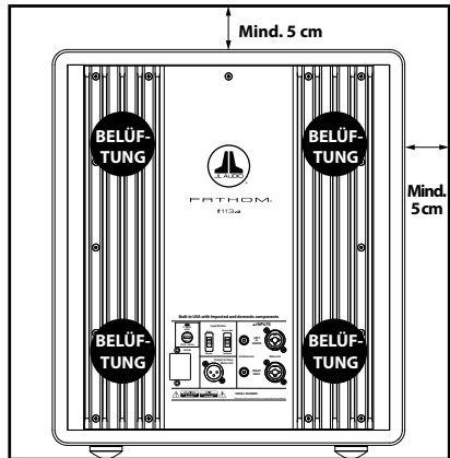
Rückansicht bei Gehäuseeinbau (f110, f112, f113):
