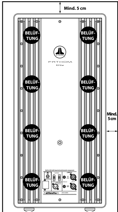
Rückansicht bei Gehäuseeinbau (f212):
