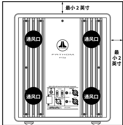
机柜安装背面视图 (f110、f112、f113) :
